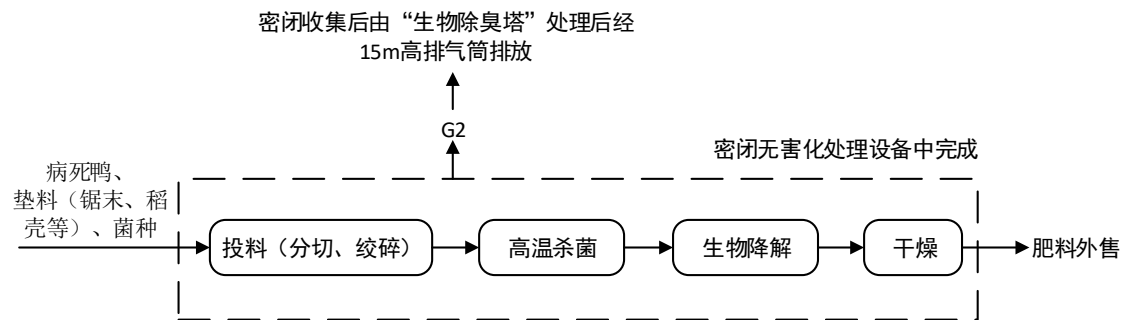
图2.4-2 病死鸭无害化处理工艺流程及产污环节图
