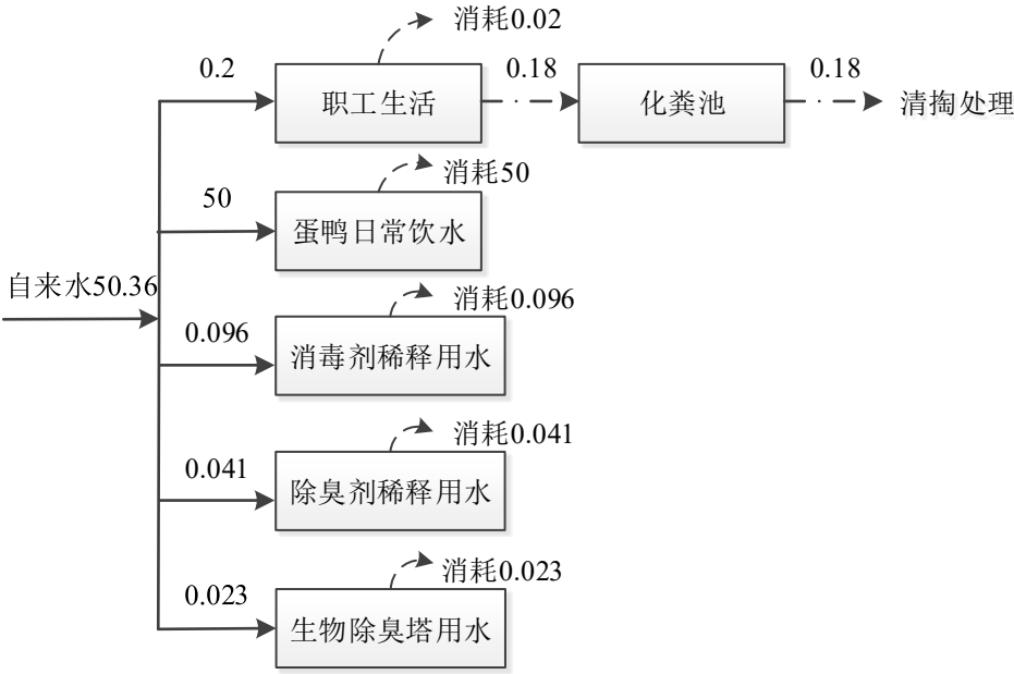
图2.2-1 本项目冬季水平衡图 m³/d
