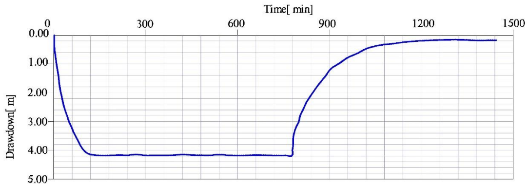
图 3.7-2 Q2 井抽水实验降深--时间曲线图
