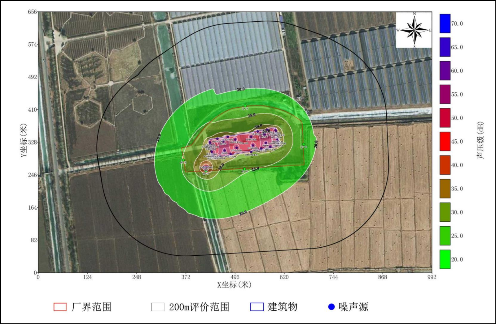
图 5.3-2 本项目噪声等声级线图（夜间）
