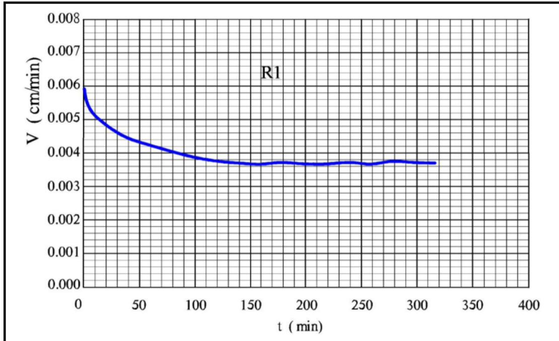
图 3.7-3 R1 入渗速率历时曲线图
