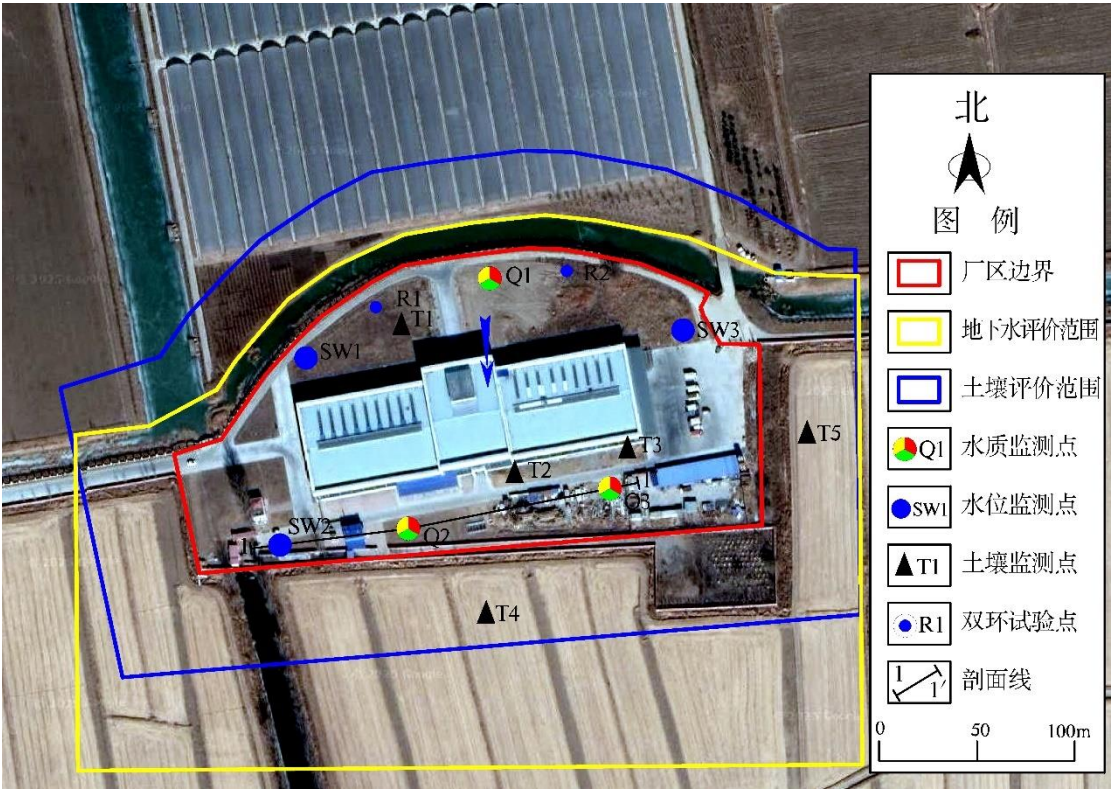
图 3.4-1 养殖区调查评价区主要实物工作布置图
