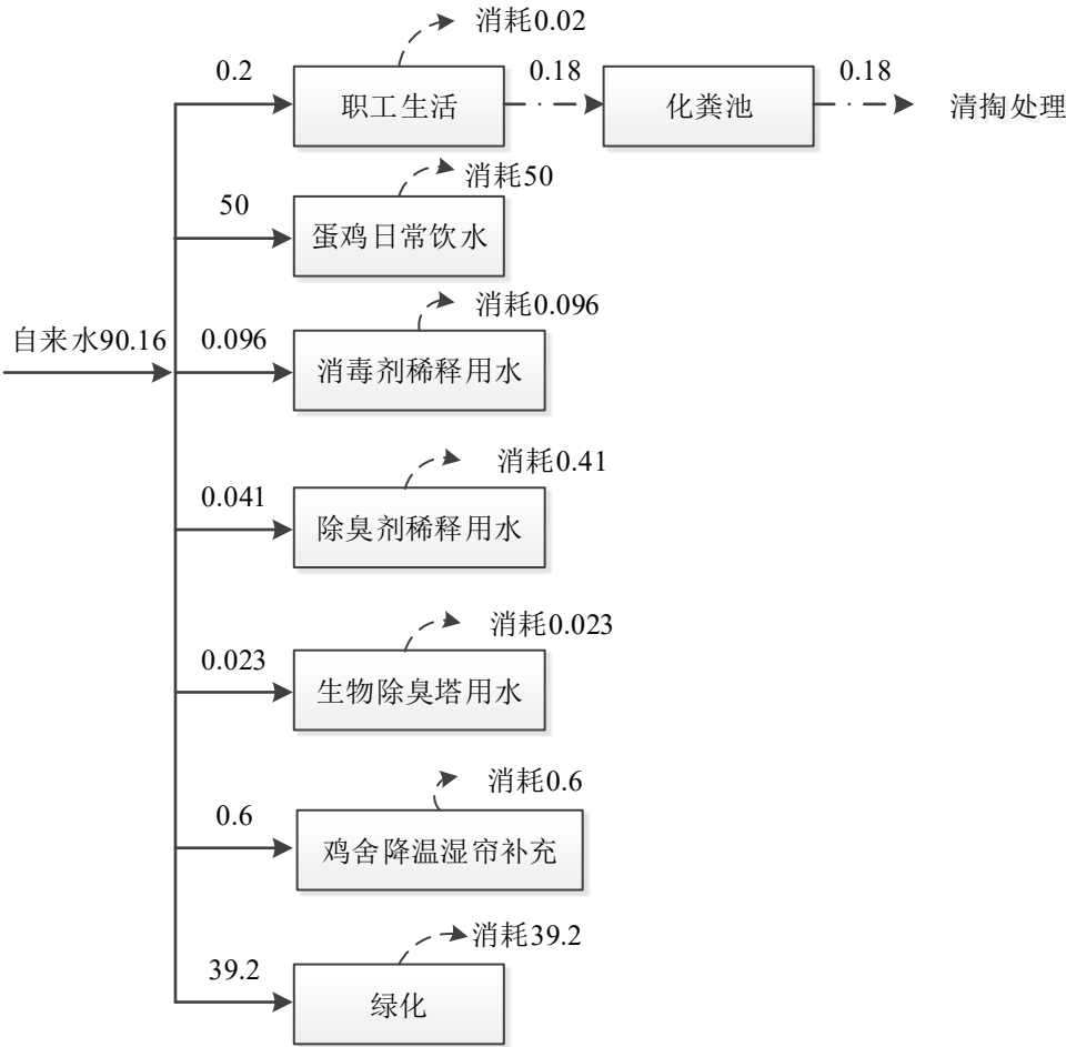
图2.2-1 本项目冬季水平衡图 m³/d
