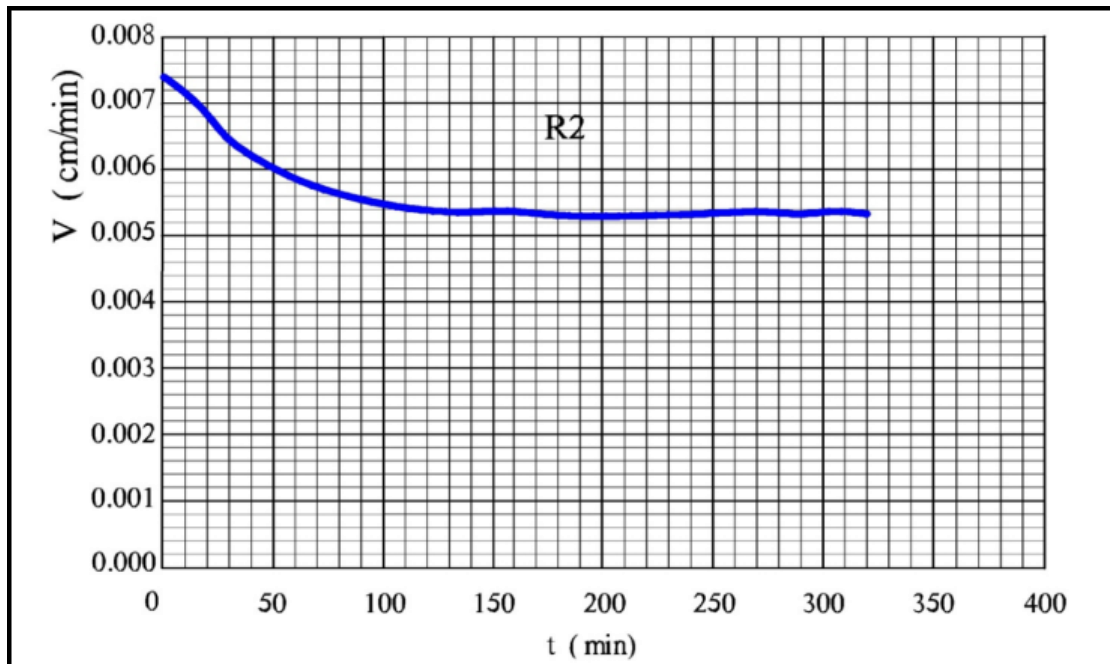
图 3.7-4 R2 入渗速率历时曲线图
