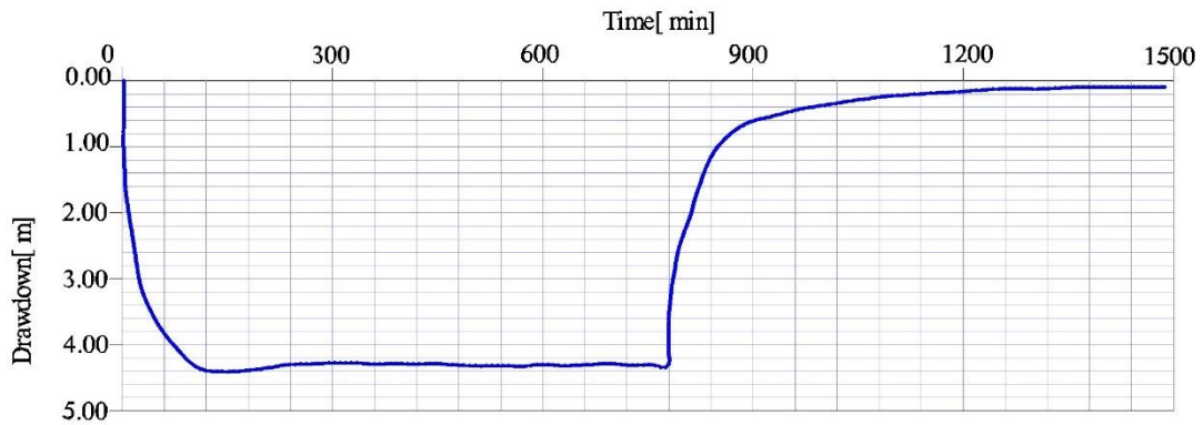
图 3.7-1 Q1 井抽水实验降深--时间曲线图
