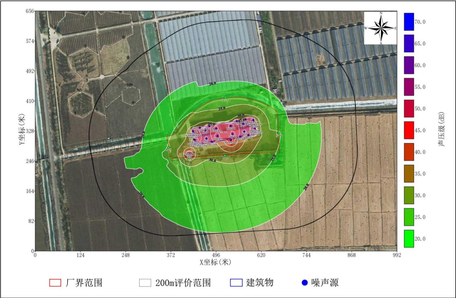
图 5.3-1 本项目噪声等声级线图（昼间）
